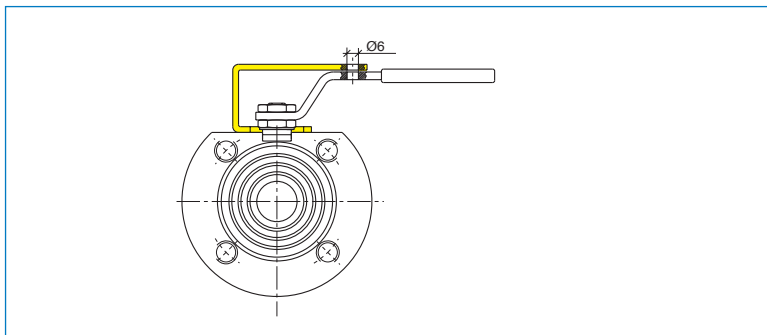
Staffa per sistema di lucchettaggio (lucchetto escluso) - Locking handle device (lockpad excluded) - Dispositif de blocage (système de cadenassage exclu) Blockiervorrichtung (Hängeschloss ausgeschlossen) - Dispositivo de bloqueo (candado no incluido)
