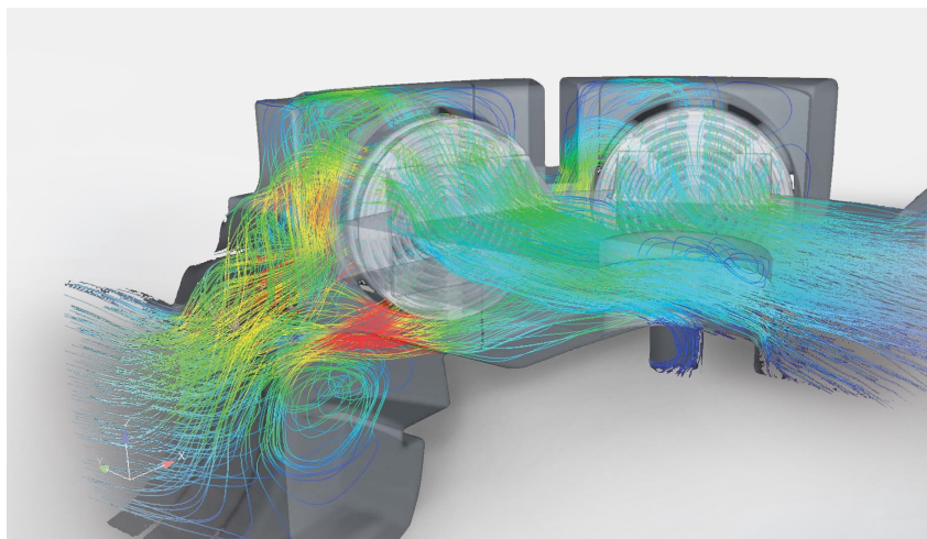
Fluid-dynamic evaluation
